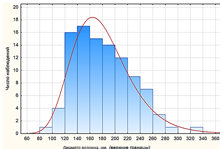
Рисунок 5 – Гистограммы логнормального распределения диаметров волокон из раствора ПВС с добавлением 7 % глицерина
