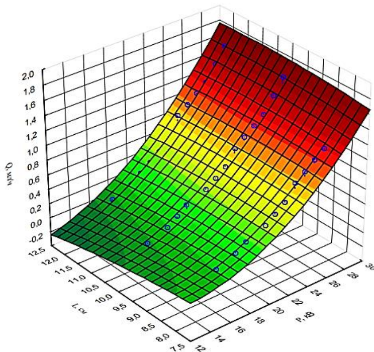
Рисунок 3 – Зависимость расхода прядильного раствора от электрического потенциала эмиттера и расстояния от эмиттера до коллектора
