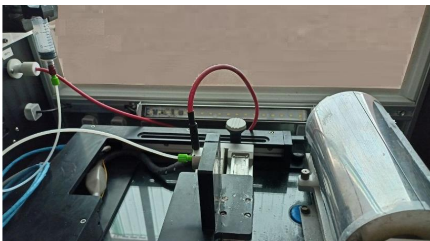
Рисунок 1 – Внешний вид рабочей зоны установки Fluidnatek LE-50
