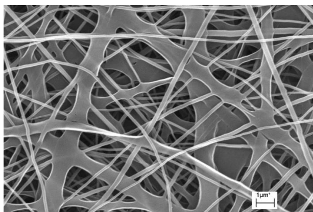
Рисунок 7 – Изображение структуры гемостатической пленки (×15000)
