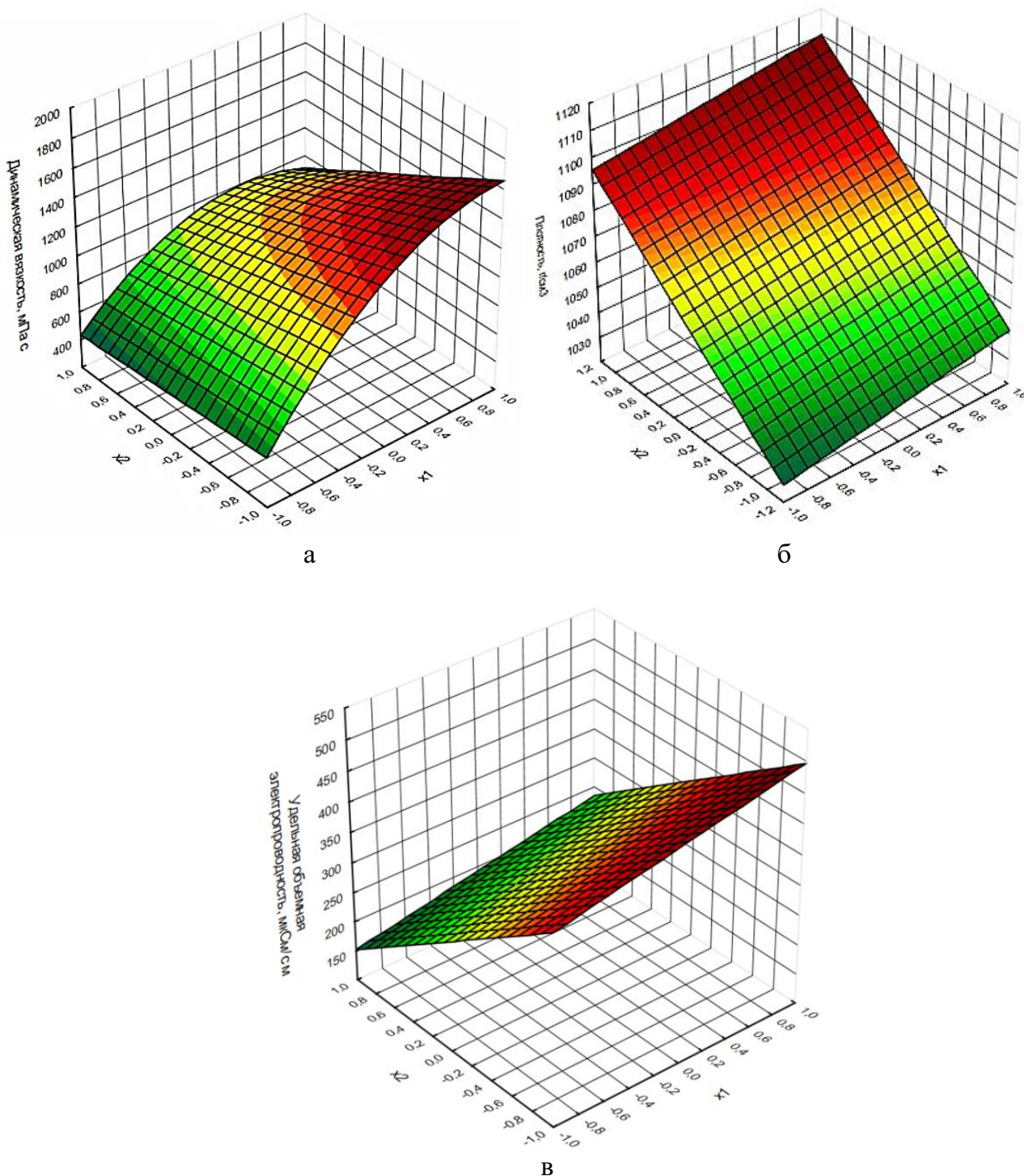
Рисунок 2 – Зависимости свойств растворов от входных факторов эксперимента
