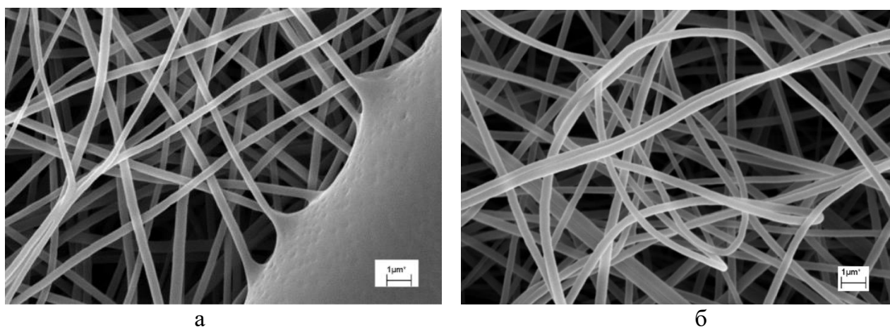
Рисунок 8 – Изображения структуры нановолокнистых материалов на основе поливинилового спирта (×15000)
