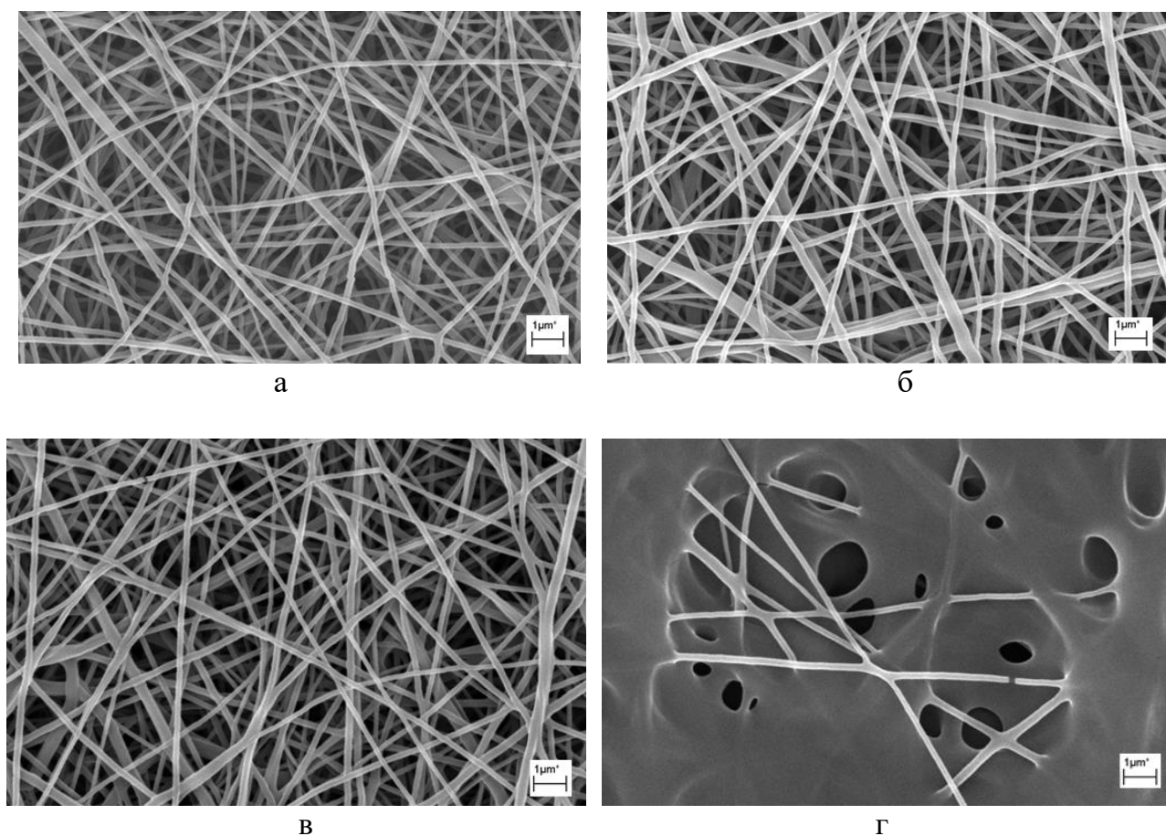
Рисунок 4 – Изображения нановолокнистых материалов ( \times 15000 ) при электроформовании из 14%-го раствора ПВС с добавлением глицерина
